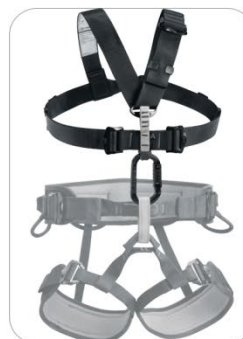
TORSE CHEST'AIR ET HARNAIS CUISSARD FALCON FORMANT UN HARNAIS ANTICHUTE
